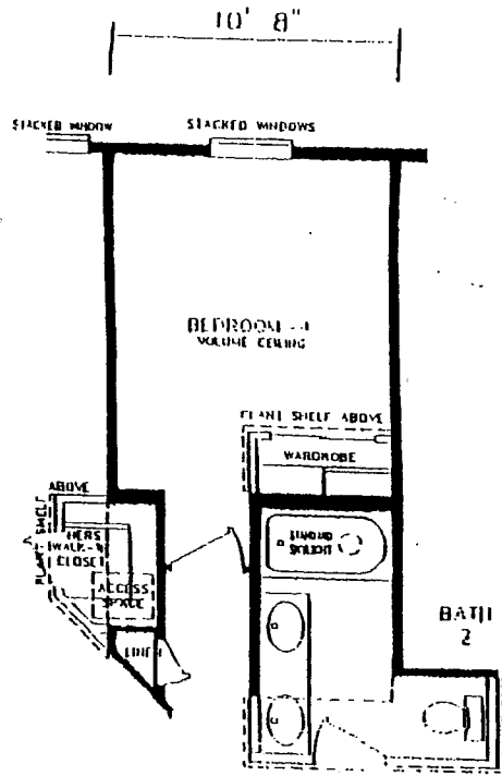
OPTIONAL BEDROOM - 1
